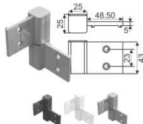
Bisagra para puerta batiente Eurovent Serie 70
